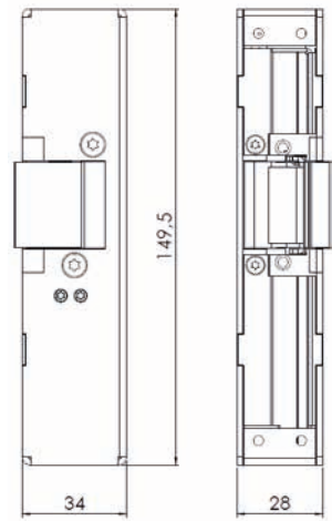
Måttskiss STEP 60 Silent.
