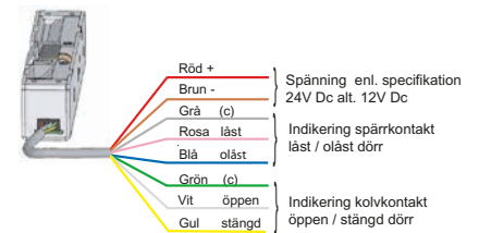
Kopplingsschema med kolvkontakt.
